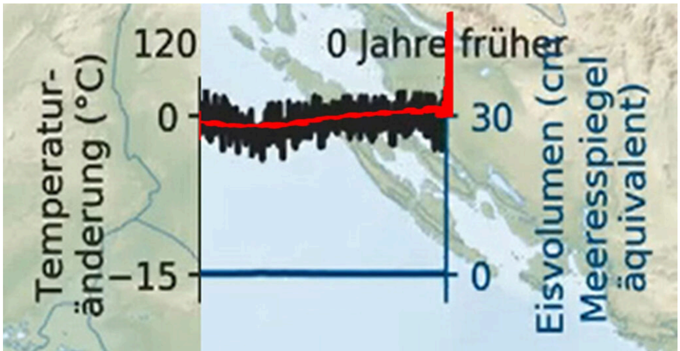
Bild 11. Eine genauere Betrachtung des Zeitraums der letzten ca. 10.250 Jahre – also lange nach Ende der letzten Kaltzeit und bis zum Beginn des Industriezeitalters (Grafik: Autor +Screenshot aus https://www.youtube.com/watch?v=TXzExbdHuDM )
