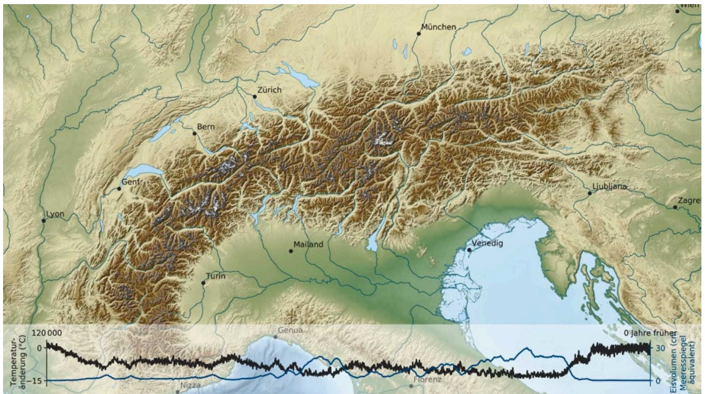
Bild 4. Die heutige Vergletscherung der Alpen. Nennenswerte Gletscherbedeckungen sind bei diesem Masstab lediglich im Umfeld des Mont Blanc sowie der Berner Alpen zu erkennen. Am unteren Bildrand sind in Schwarz die Temperaturunterschiede zum heutigen Niveau (linke Skalenachse) sowie auf der rechten Skala das Eisvolumen in cm Meeresspiegel-Aequivalent zu erkennen
