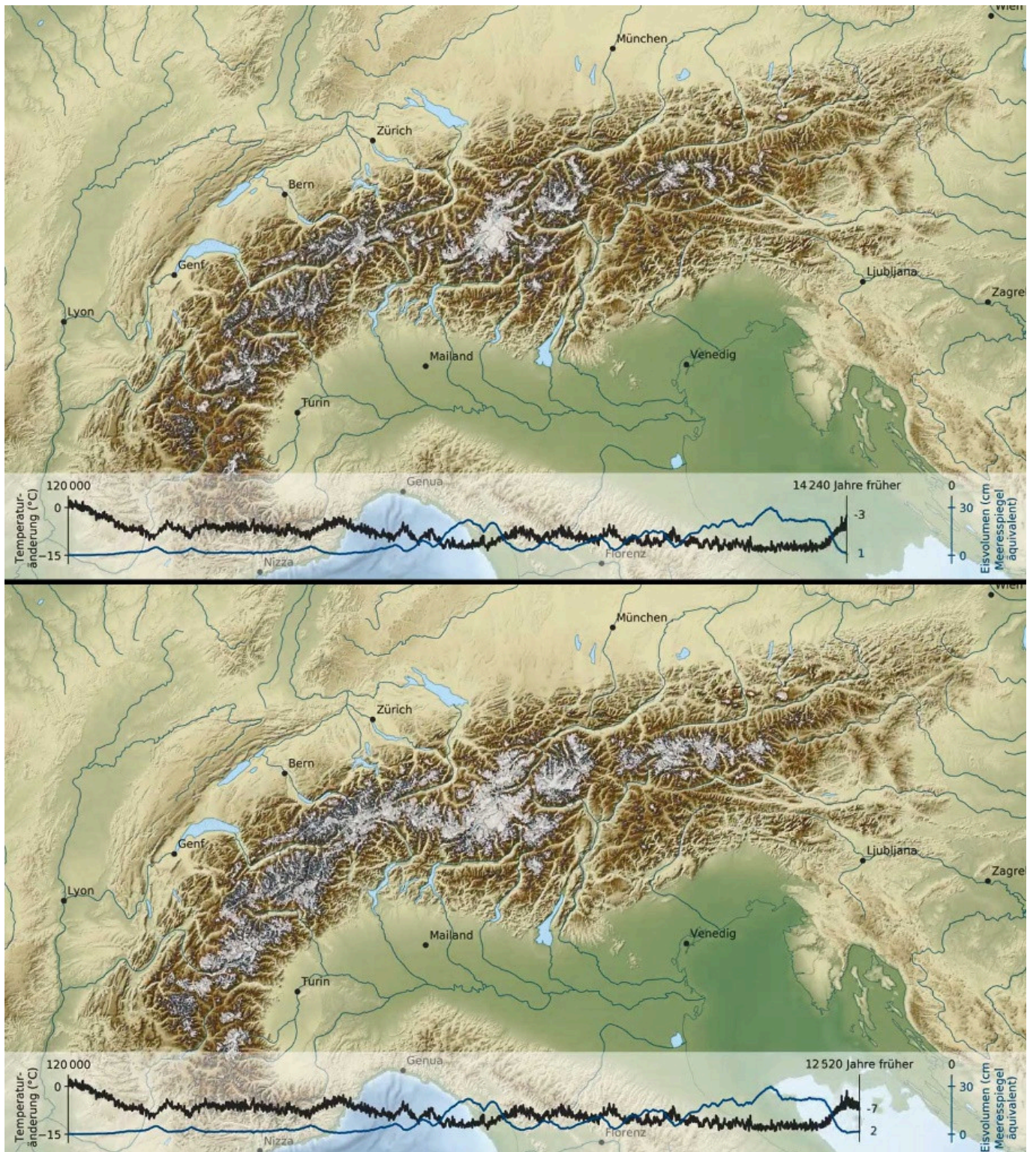
Bild 9. Auch das Ende der Kaltzeit verlief alles andere als gleichmässig. Nach einem bereits recht weitgehenden Abschmelzen der Gletscher um das Jahr 14.240 herum
