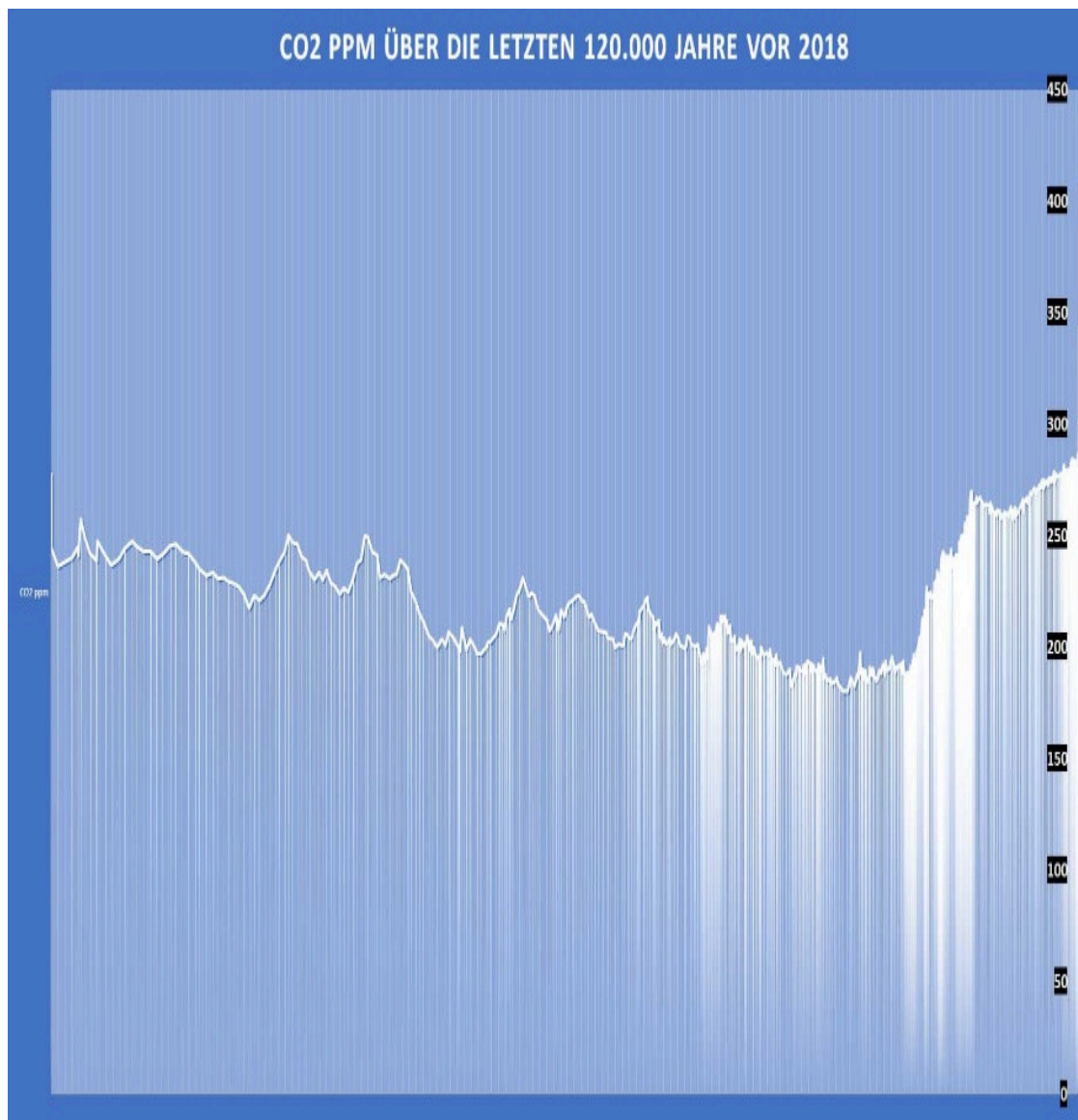
Bild 3. Der von der offiziellen Klimawissenschaft ermittelte Verlauf des CO 2 -Gehalts in der Atmosphäre in den letzten 120.000 Jahren. Erst ganz am Ende der steile Anstieg zu den heutigen Werten, der in den Alpen ein „Gletschersterben“ verursachen soll (Grafik: Autor, mit Daten von Our World in Data 6) )
