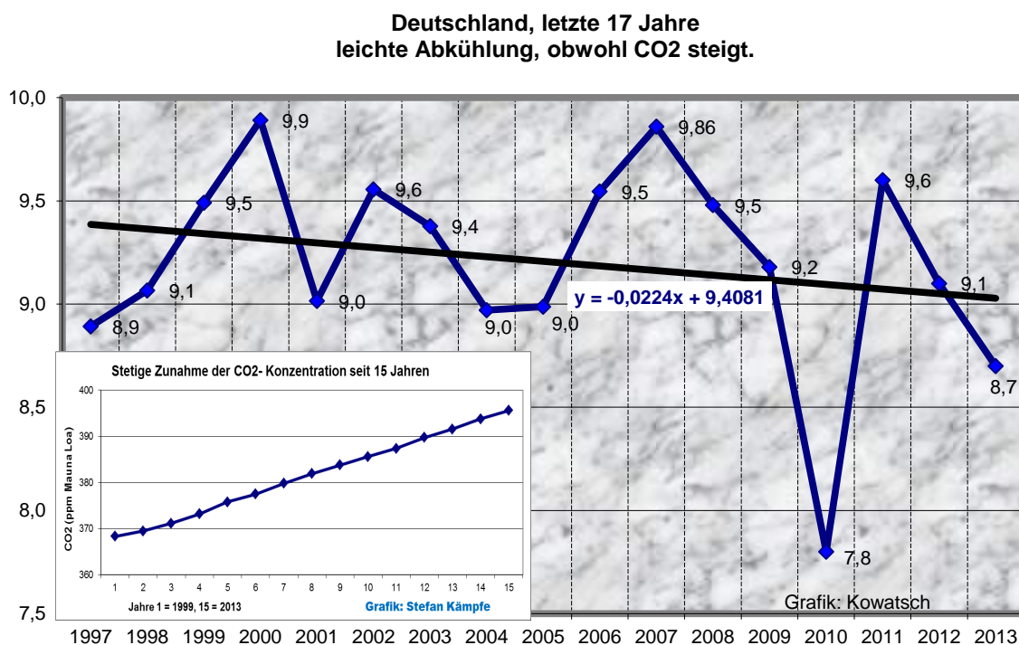
Abb. 2: Temperaturverlauf in Deutschland seit 17 Jahren
