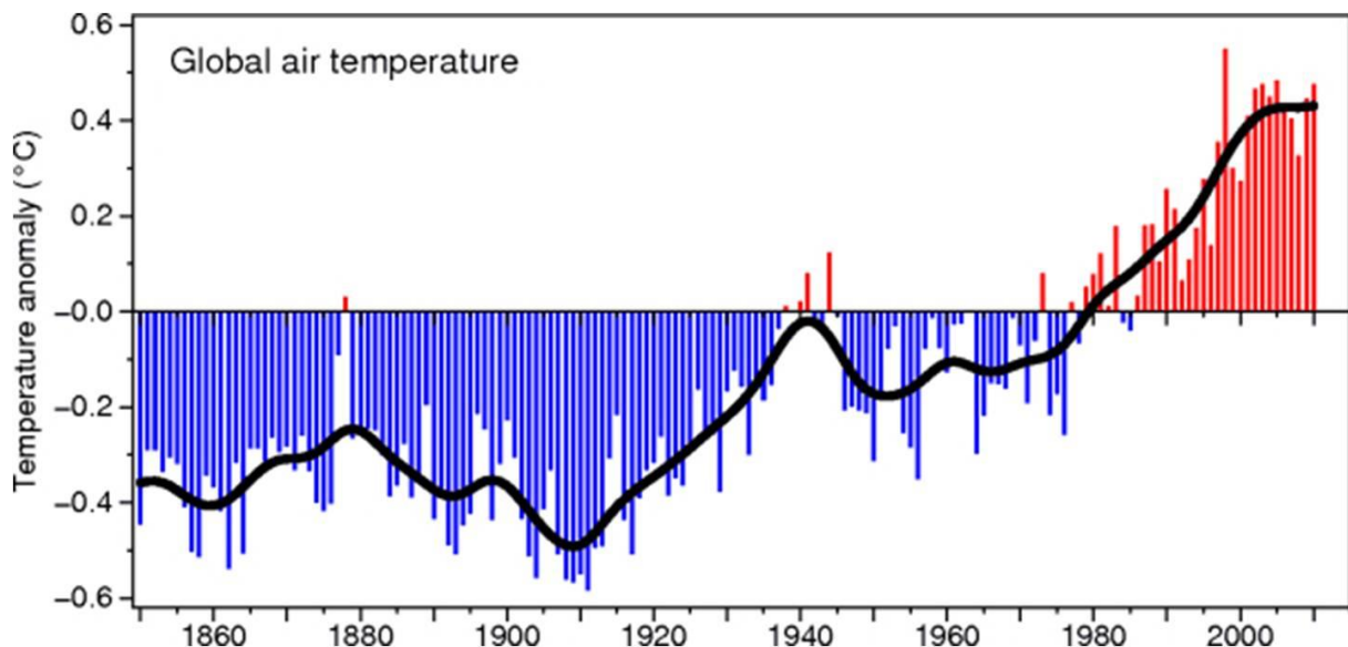
Abb. 1: Globaltemperaturverlauf seit 1850
